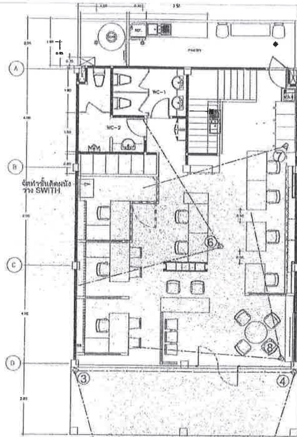
1st FL. LAY OUT PLAN สาขาหาดใหญ่
