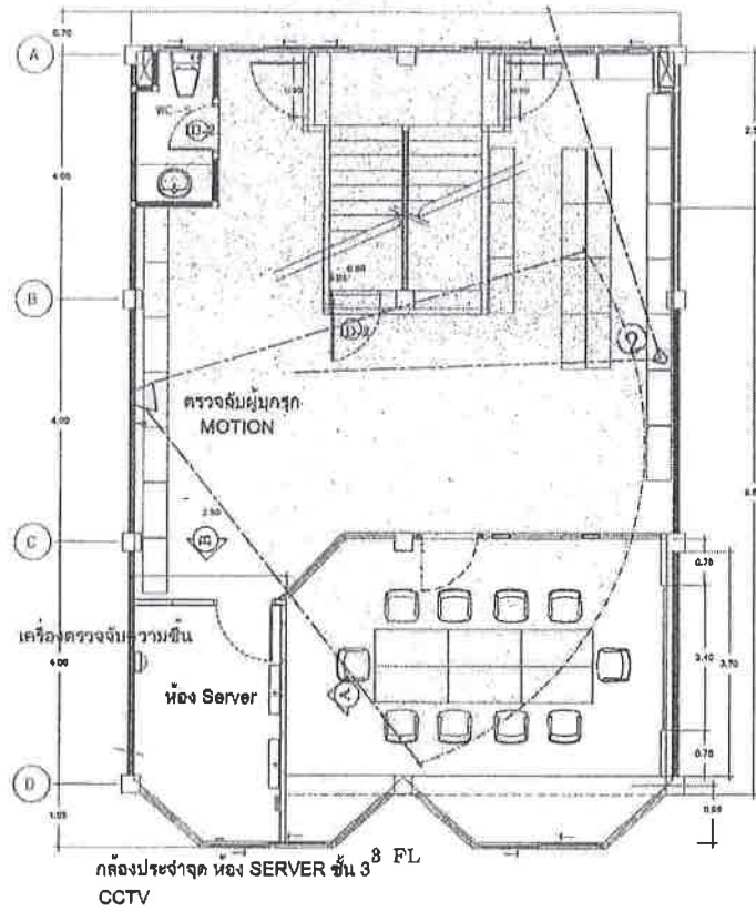
3rd FL LAY OUT PLAN สาขา หาดใหญ่
